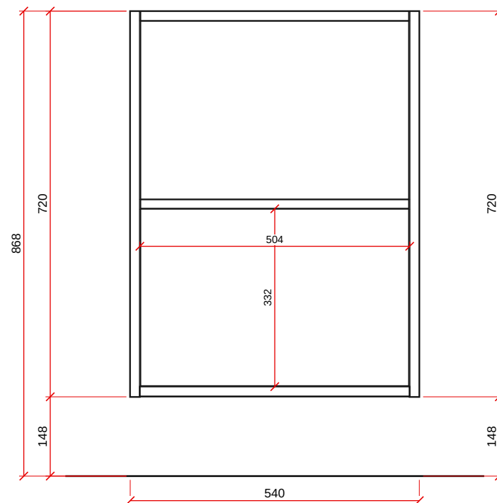
VISTA B - ESC. 1:10
